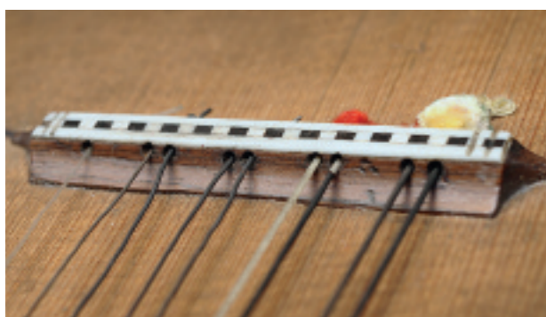
Abb. 206 Terzgitarre TieWV 111: Steg mit der originalen Saitendisposition – ehemals wohl aller Gitarren Tielkes
